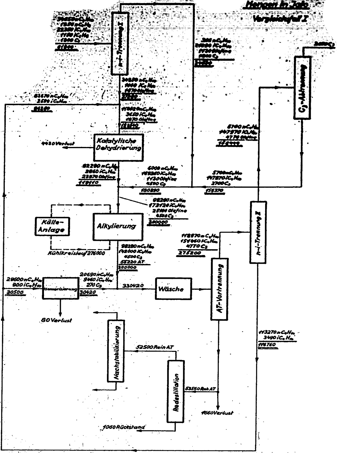
Mengenschema zur AT-Anlage mit katalytischer Dehydrierung 60000 Tons C 2 Einsatz
