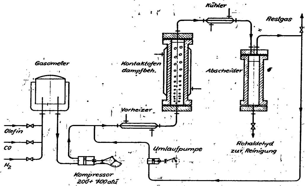
Schema der Oxo-Anlage zur Herstellung von Propionaldehyd und Isobutylaldehyd aus Äthylen bzw. Propylen
