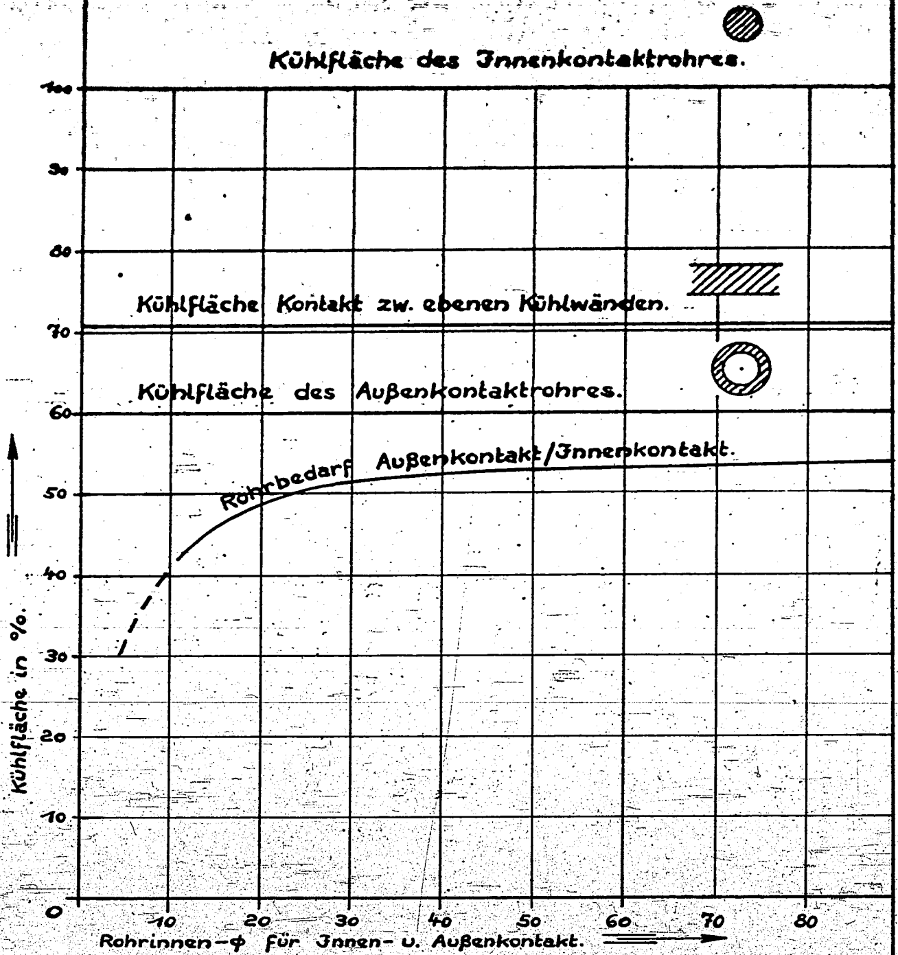
Abbildung Der Kühlflächenbedarf bei verschiedenen gefüllten Reaktionsröhren.
