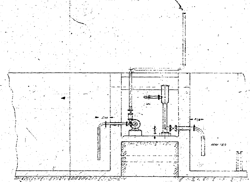
Schnitt C-D
