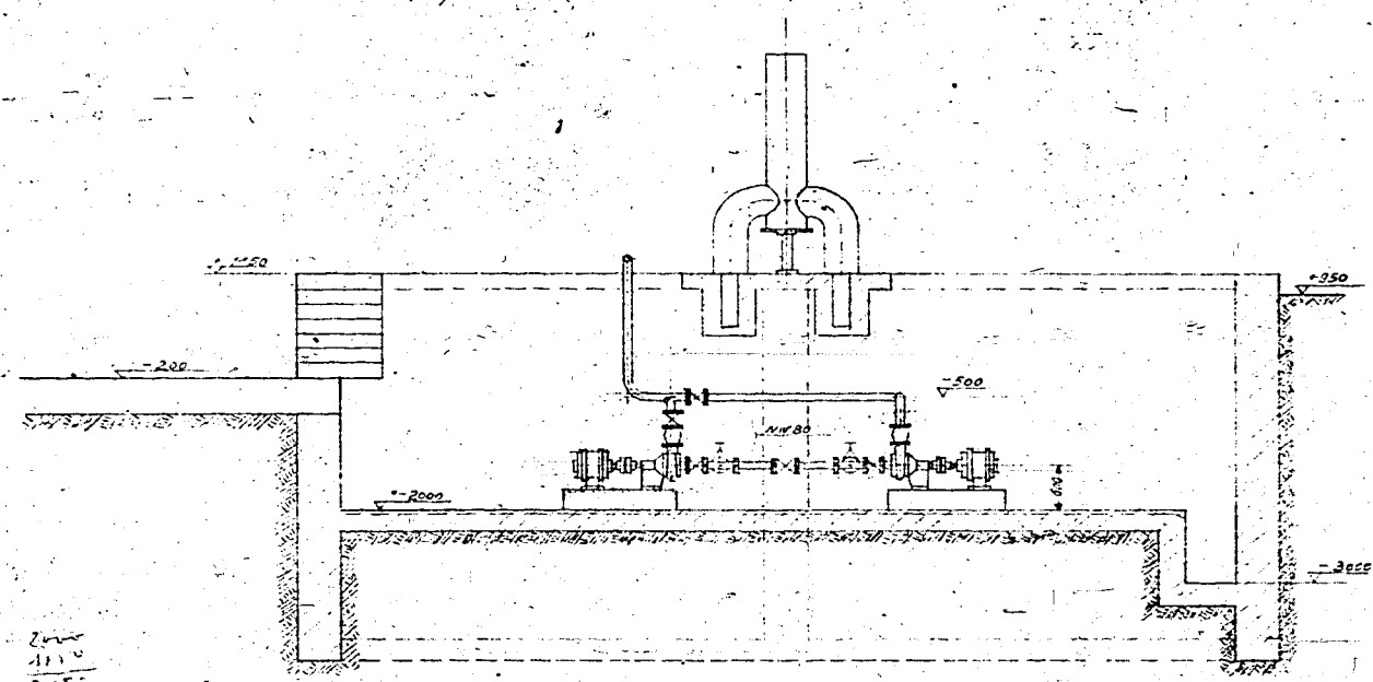
Schnitt A-B
