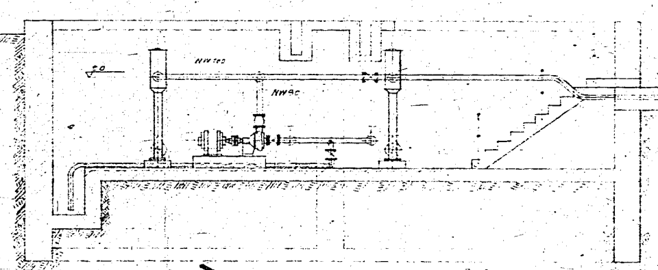
Schnitt E-F
