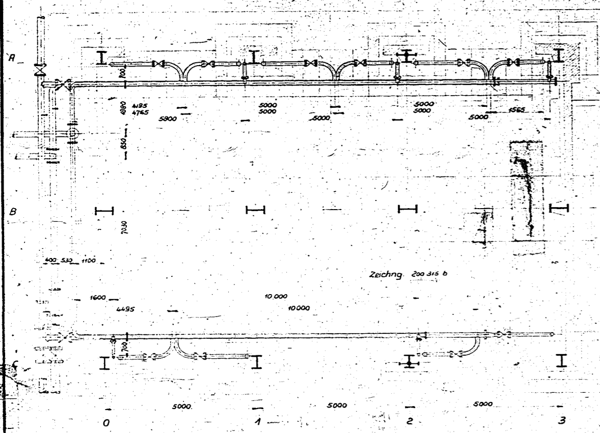
Grundriss 10
