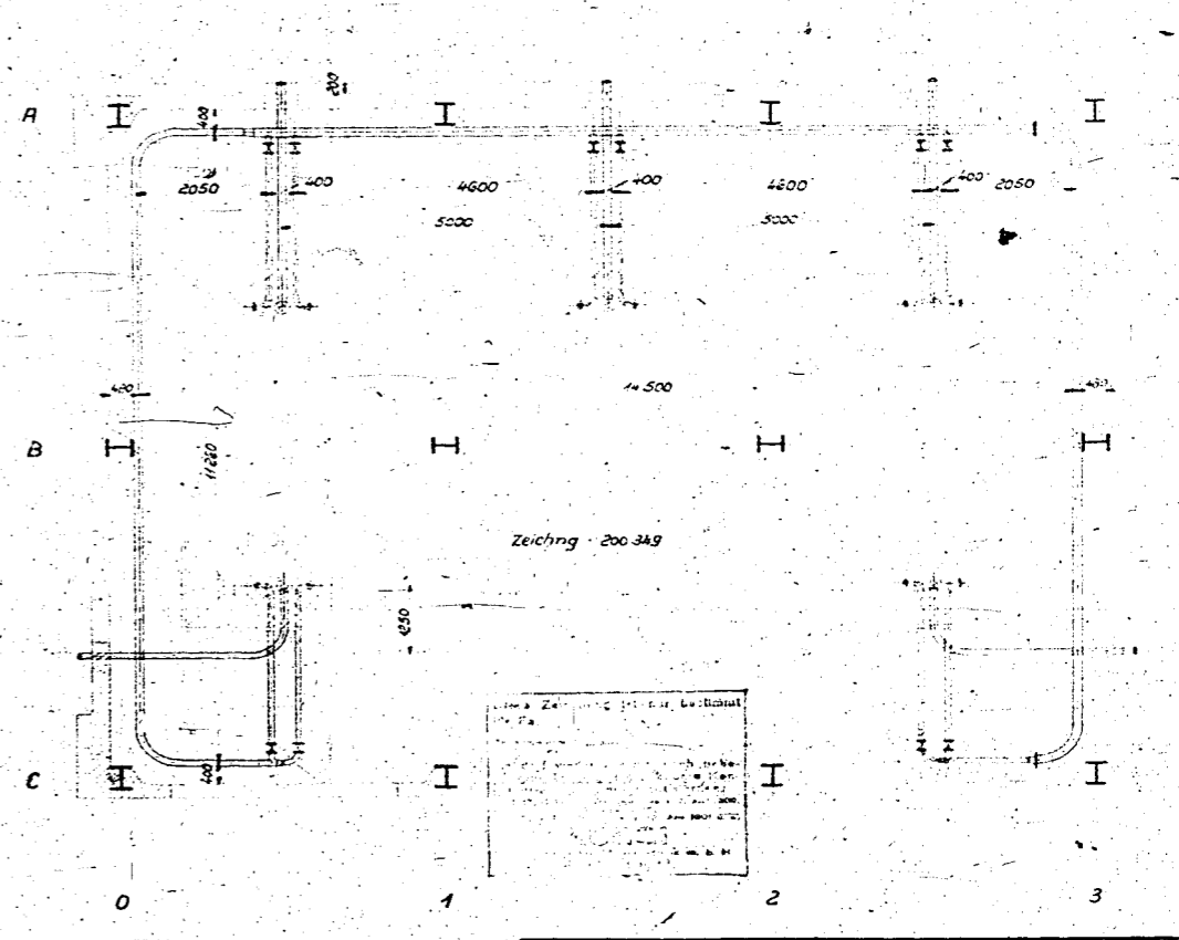
Schnitt in Höhe + 17 310
