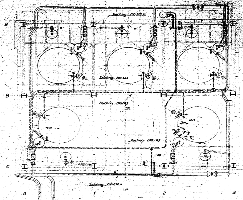
Bühne + 11 000
