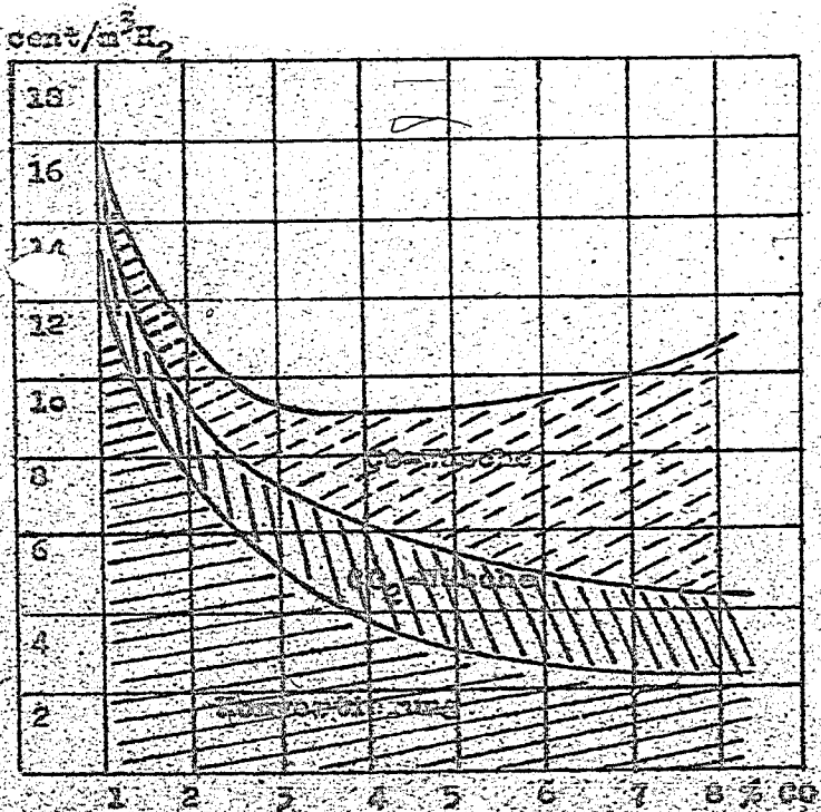
Abb.3. Wassergas No.1. Kosten der Kohlevergasung + CO 2 -Wäsche + CO-Wäsche. Verschiedene CO-Gehalte nach der Kohlevergasung (Energie + Dampf).
