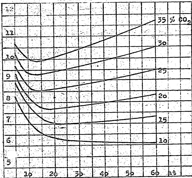
Abb.1. Energieverbrauch bei der CO 2 -Wäsche für verschiedene CO 2 -Gehalte im Ausgangsgas in Abhängigkeit vom Waschdruck.
