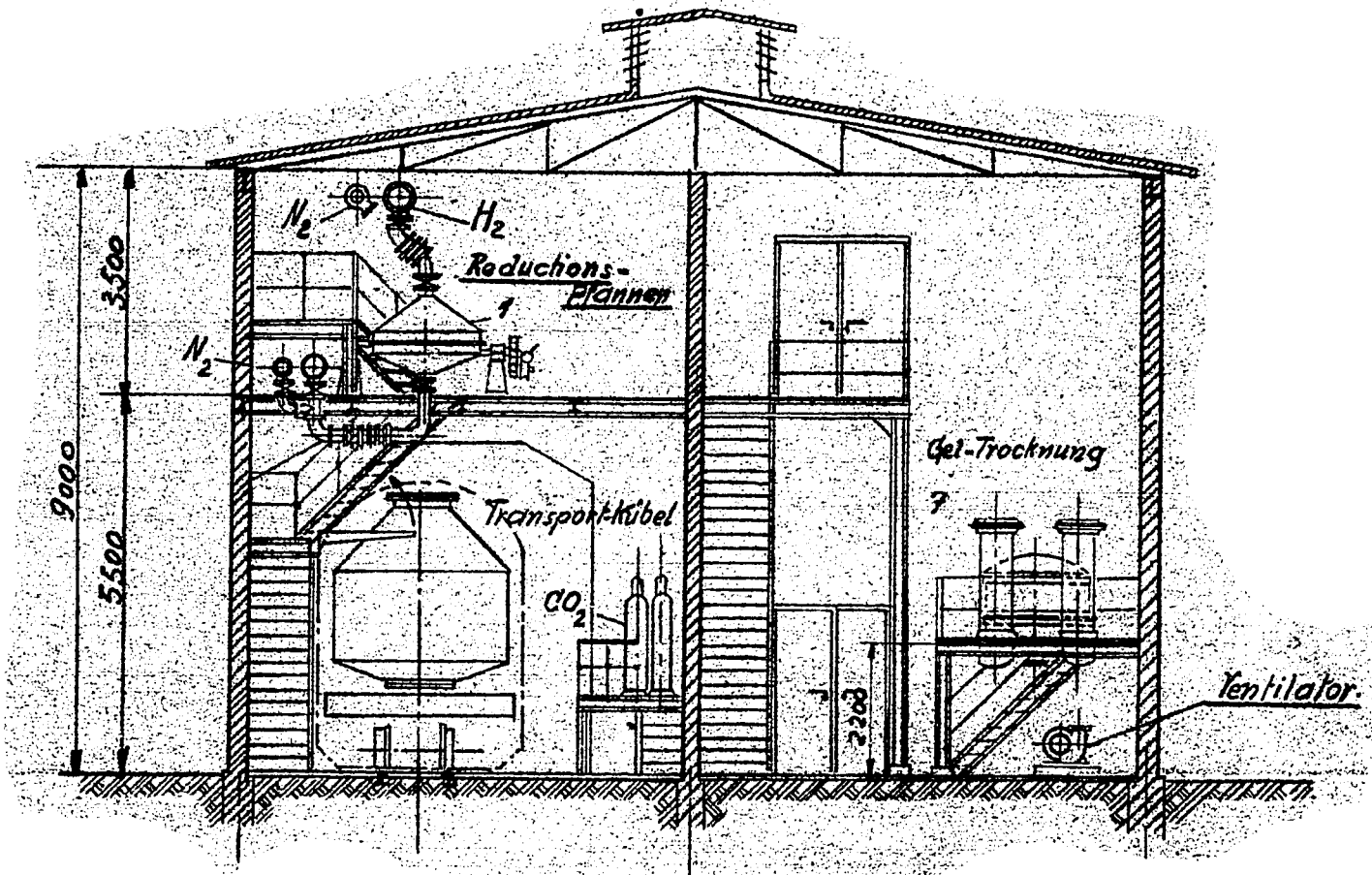
Schnitt C-II section
