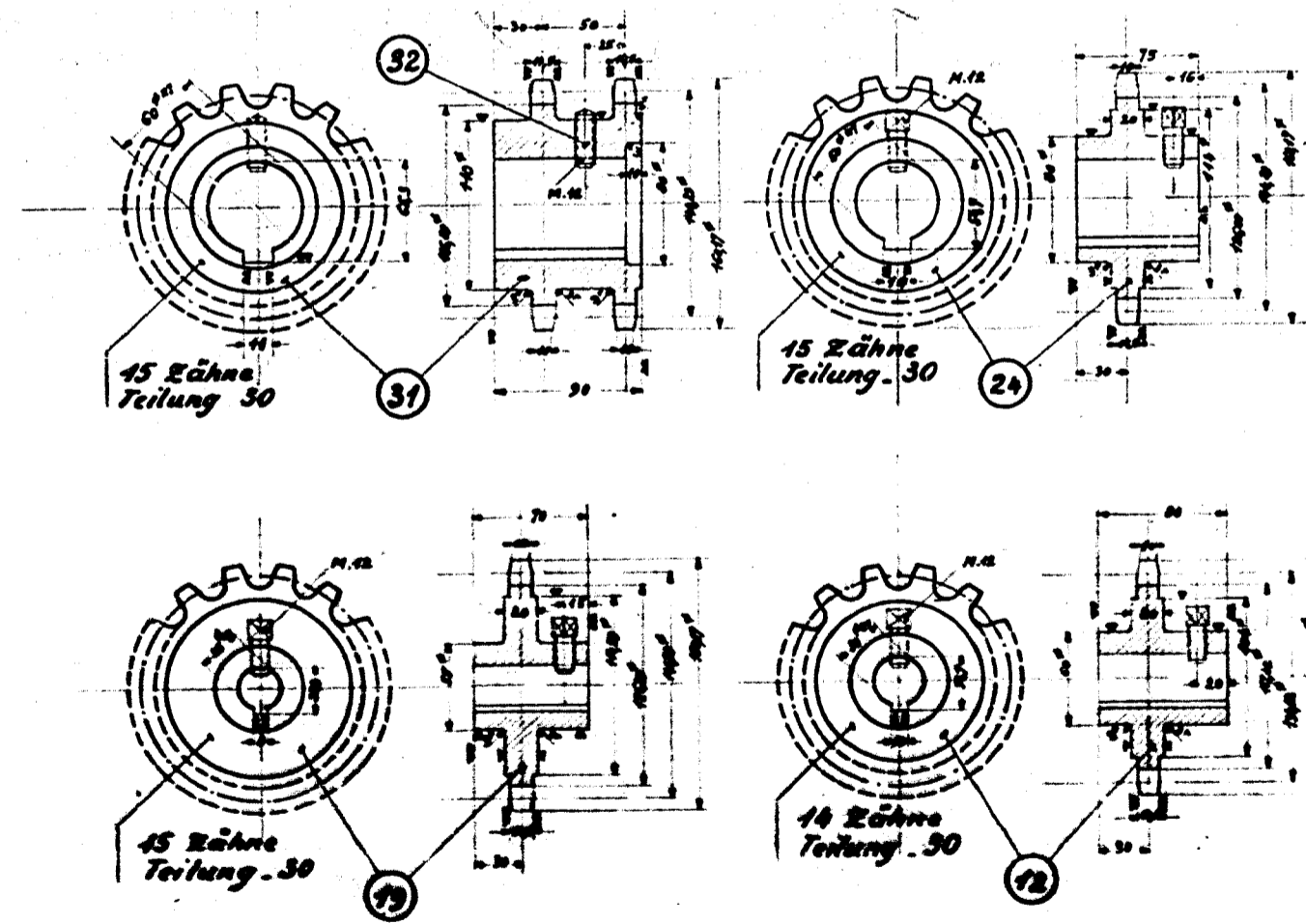
Maßstab: 1:25
