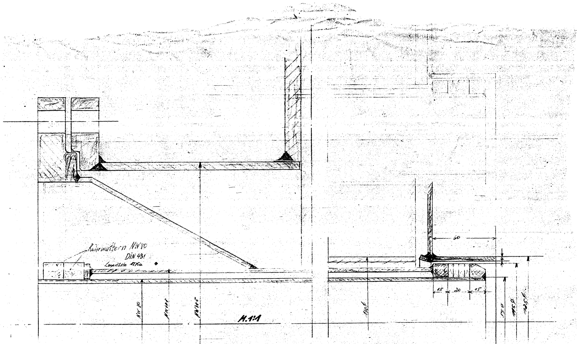
Eingangsstutzen für untere Spülrinne (Reg.-Teil)
