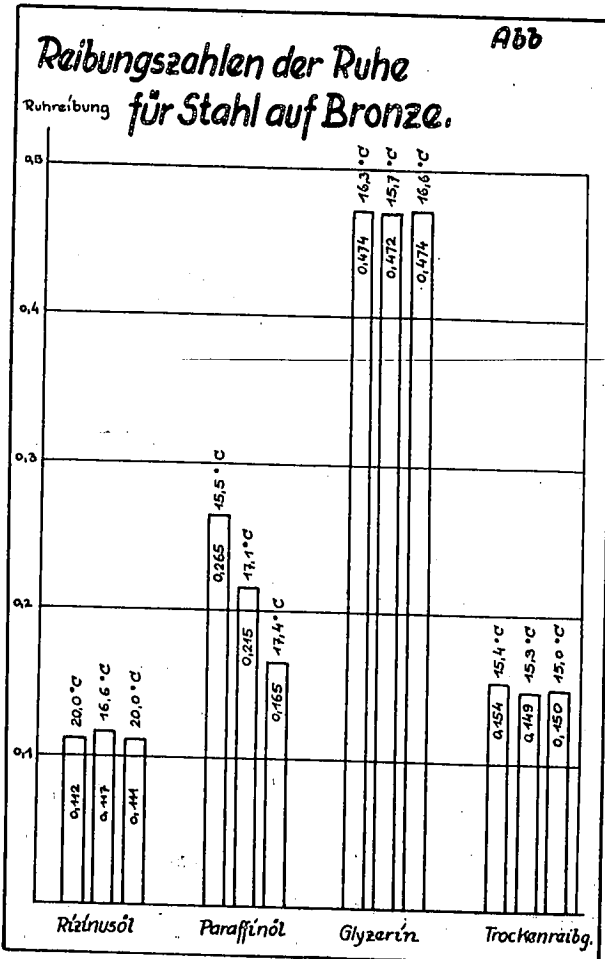
Abb.1a: Reibungszahlen der Ruhe für Stahl auf Bronze.
