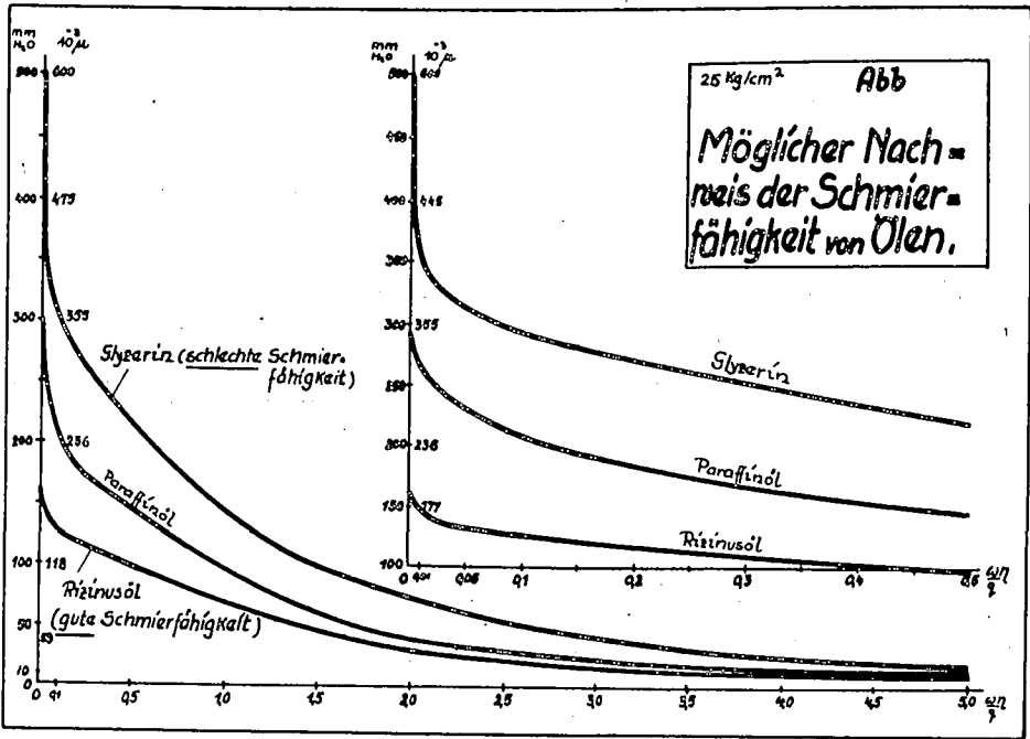
Abb.2: Möglicher Nachweis der Schmierfähigkeit von Ölen.
