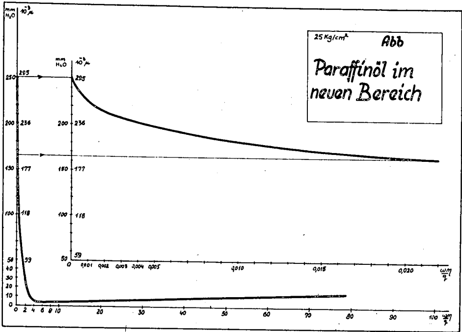
Abb.2b: Paraffinöl im neuen Bereich
