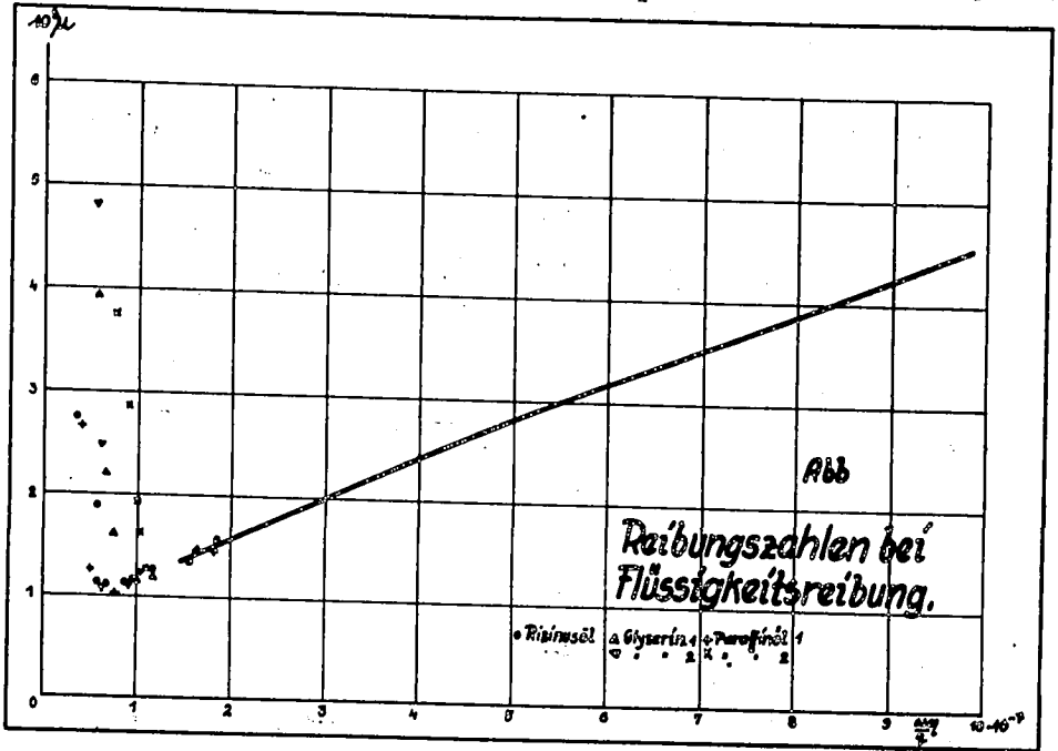
Abb. 1: Reibungszahlen bei Flüssigkeitsreibung.
