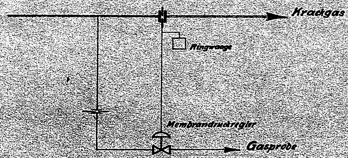
Selbsttätiger Gasprobenehmer
