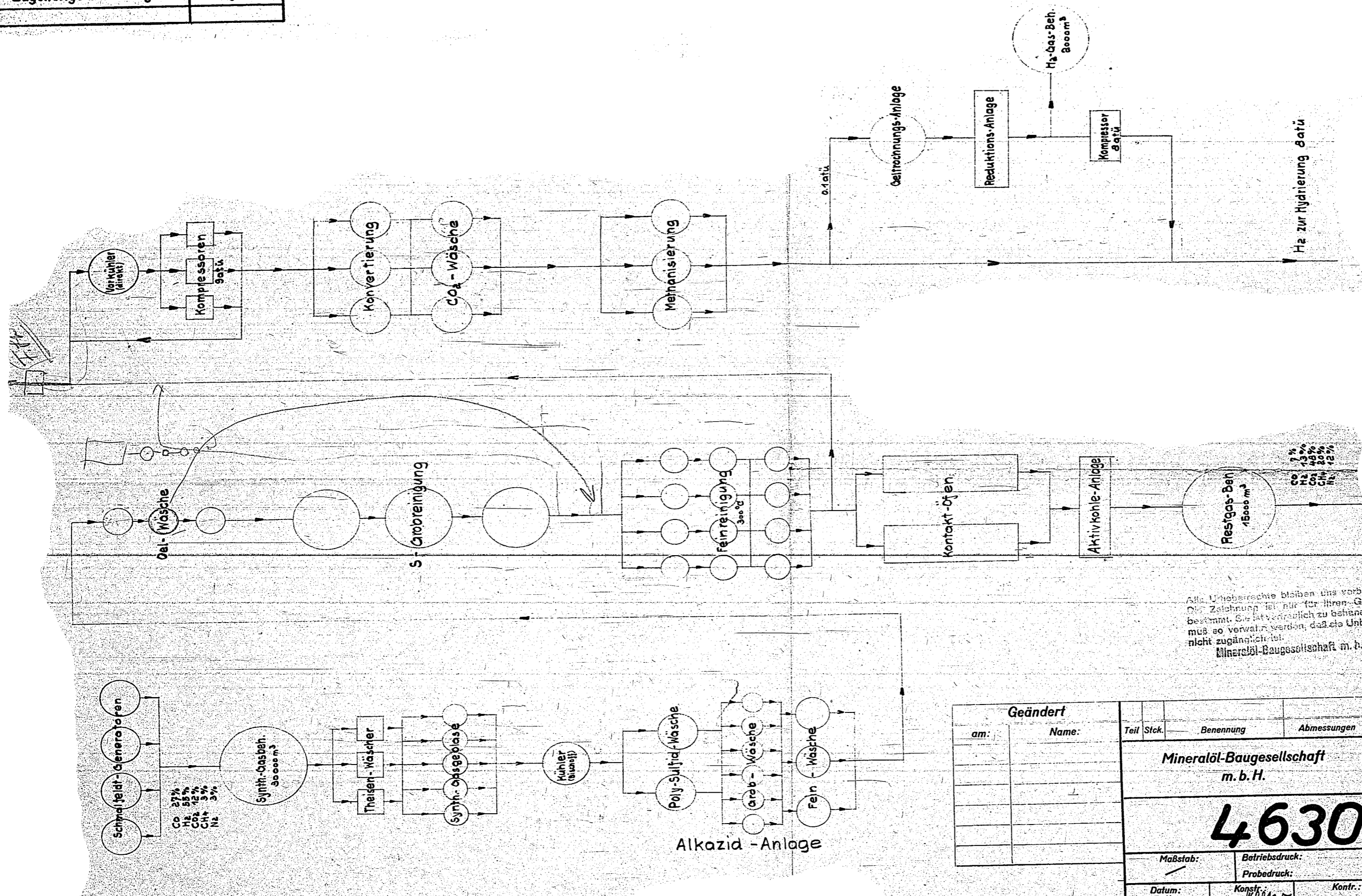
Gasschema der Benzin-Anlage Lützkendorf
