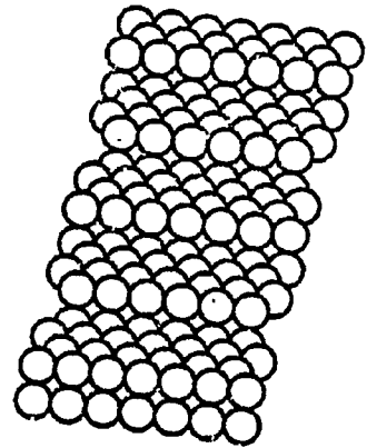
fcc (110)
