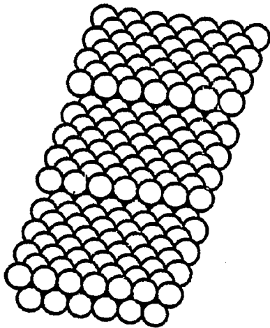
fcc (200)
